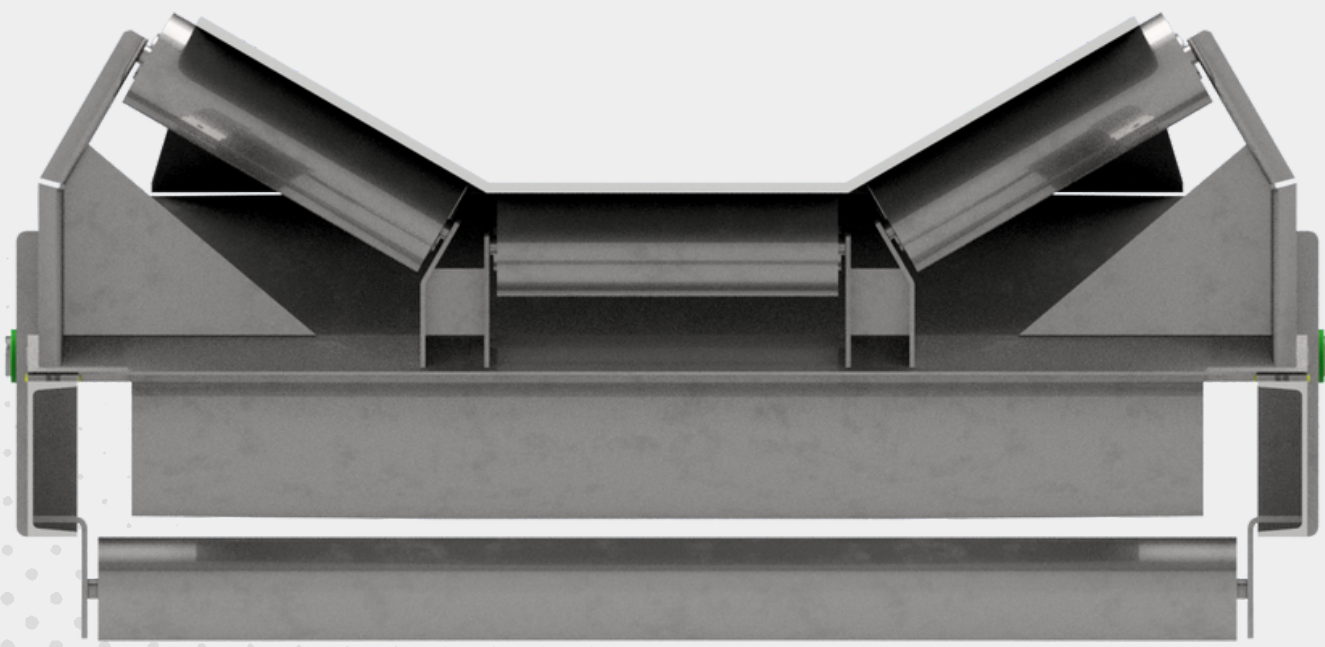
Sistema de sustentação da correia por cavaletes de carga
